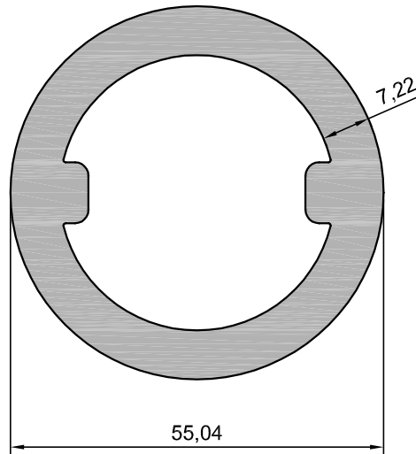
204.08 3,121 kg/m
