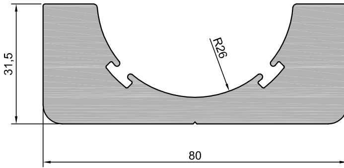
204.49 4,012 kg/m
