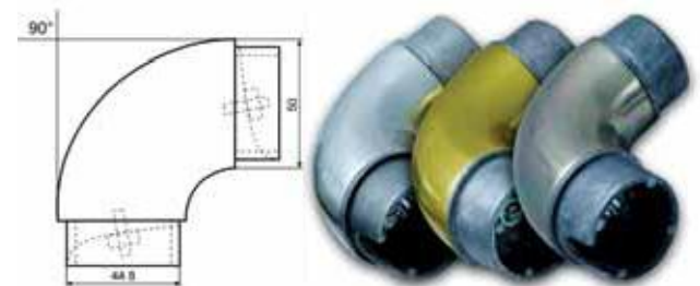
Ø 50'lik 1/4 Boş Dirsek
