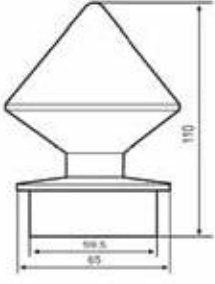
Ø 65'lik Boru Mızrak Dekorlu Tapa
