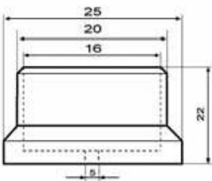
Ø 16'lik Boru Flanşı
