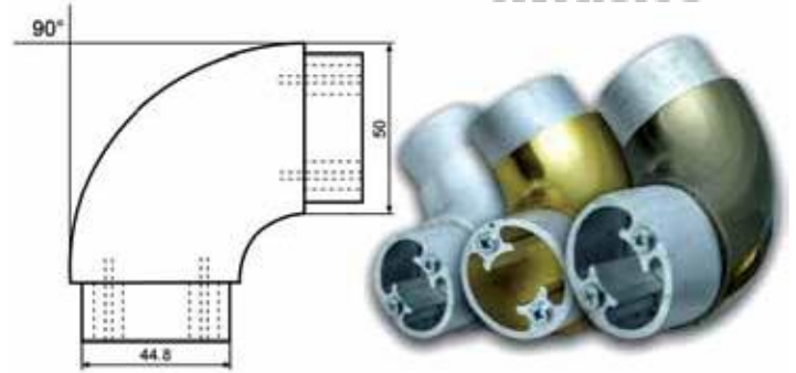
Ø 50'lik 1/4 Bağlı Dolu Dirsek
