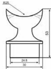
Ø 30x50 Dekorlu Sabit Mafsal
