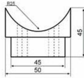
50x50 Boru Ara Bağlantı
