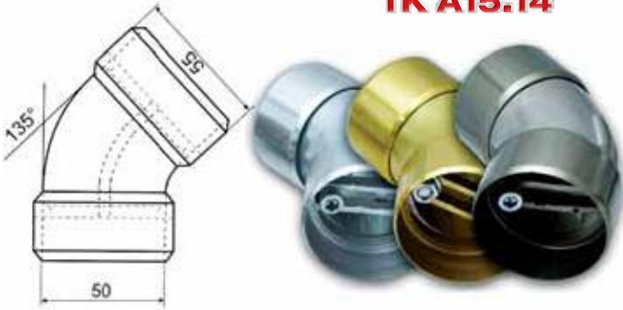
Ø 50'lik 1/8 Bilezikli Boş Dirsek
