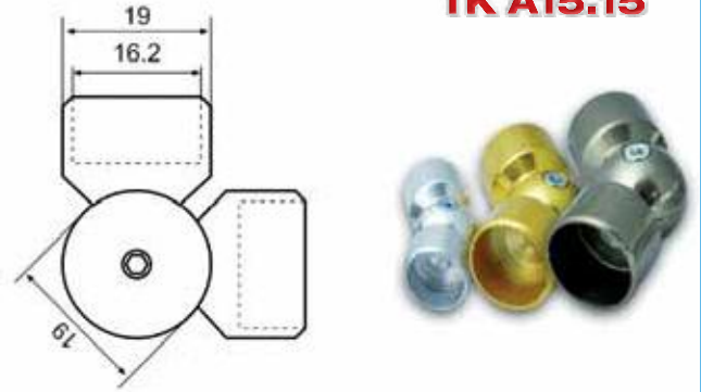
Ø 16'lik Ayarlı Küre Dirsek
