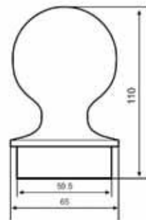
Ø 65'lık Boru Dekorlu Tapa
