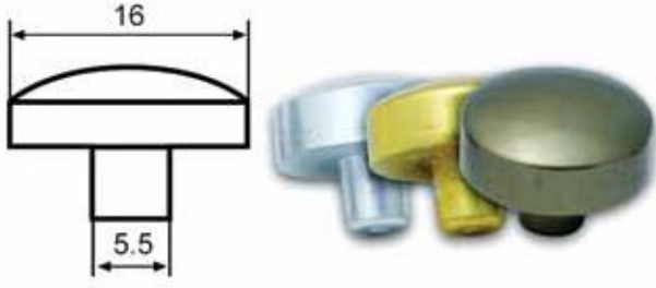
Ø 16'lık Dolu Boru Tapası
