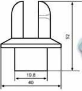
Ø 40'lik Dikme Yarıkli Tapa
