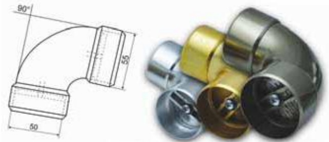
Ø 50'lik 1/4 Bilezik Dolu Dirsek
