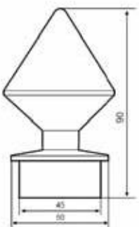
Ø 50'lık Boru Mızrak Dekorlu Tapa
