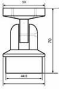
Ø 50'lik Boru Açılı Mafsal Takımı
