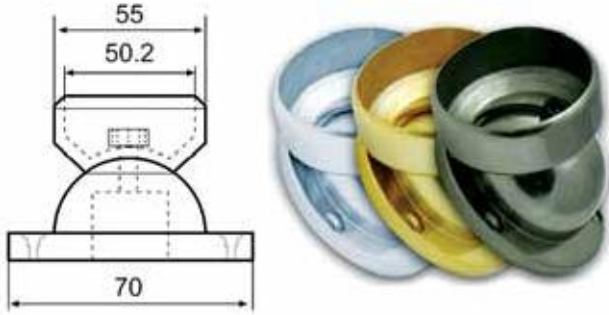
Ayarlı Küre Duvar Flanş
