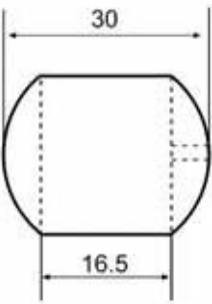
Ø 16'lık Küre Emniyet Tutamağı
