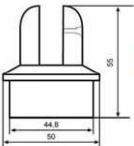
Ø 50'lik Boru Yarıkli Tapa
