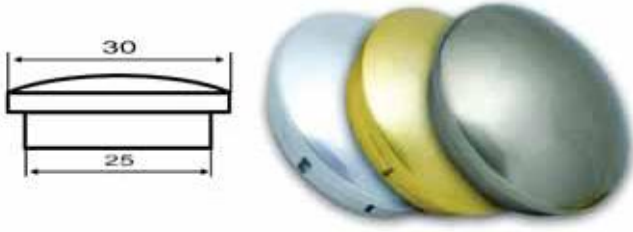
Ø 30'luk Boru Tapası
