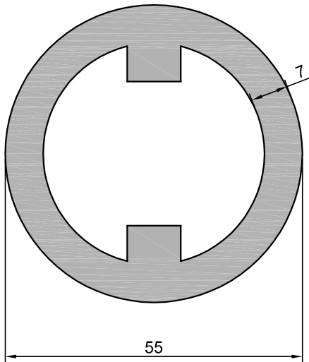
204.02 3,423 kg/m
