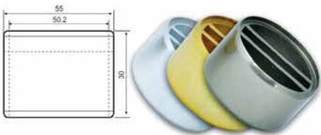
Ø 50'lik Özel Bilezik Simit Bağlantısı
