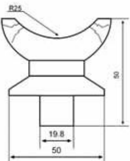
Ø 50x50 Dikme Dekorlu Sabit Mafsal
