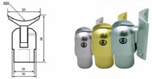
Ø 30'luk Boru Mafsal Takımı
