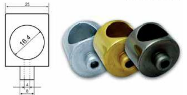
Ø 16'lık Tekli Emniyet Tutamağı
