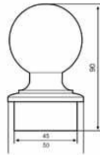
Ø 50'lık Boru Dekorlu Tapa
