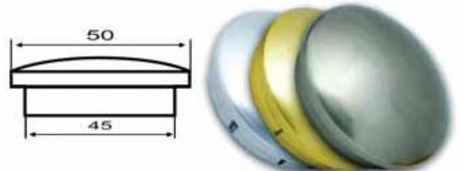
Ø 50'lık Boru Tapası
