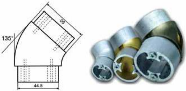
Ø 50'lik 1/8 Bağlı Dolu Dirsek
