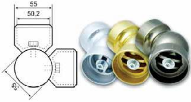
Ø 50'lik Ayarlı Küre Dirsek
