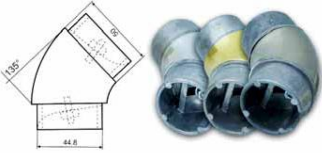
Ø 50'lik 1/8 Boş Dirsek
