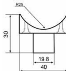
Ø 40x50 Dikme Ara Bağlantı
