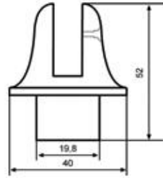
Ø 40'lik Dikme Dekorlu Yarıkli Tapa
