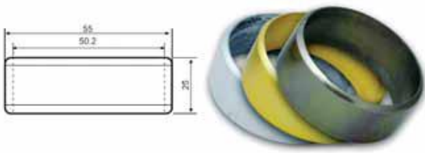
Ø 50'lik Bilezik
